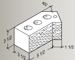
45° Dogleg
